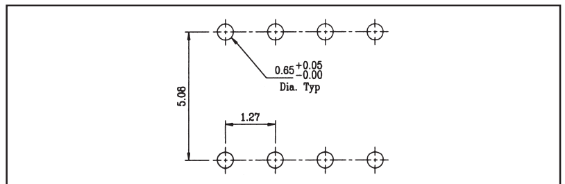
P.C.B. LAYOUT
